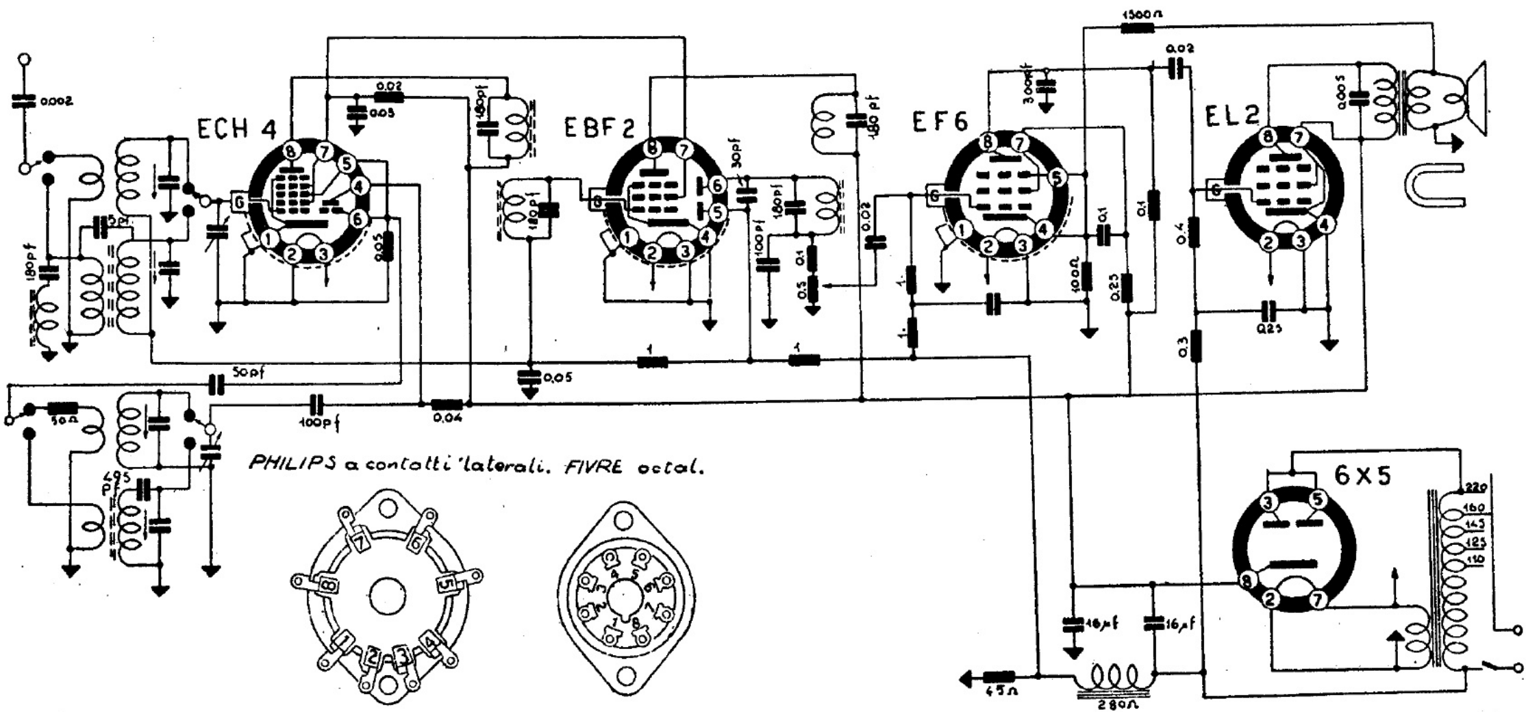
MINERVA RADIO - Mod. 455/1 - Due gamme di ricezione: da 195 a 580 m, e da 17 a 52 m. Media frequenza: 470 kc/s. Potenza d'uscita: 3 watt. Consumo: 30 watt. Altoparlante a magnete permanente. Produzione 1945-46.
